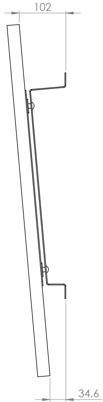
Inclinación de 5°
