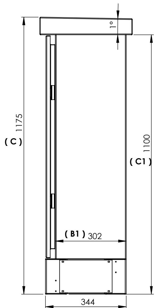
Vista Lateral
